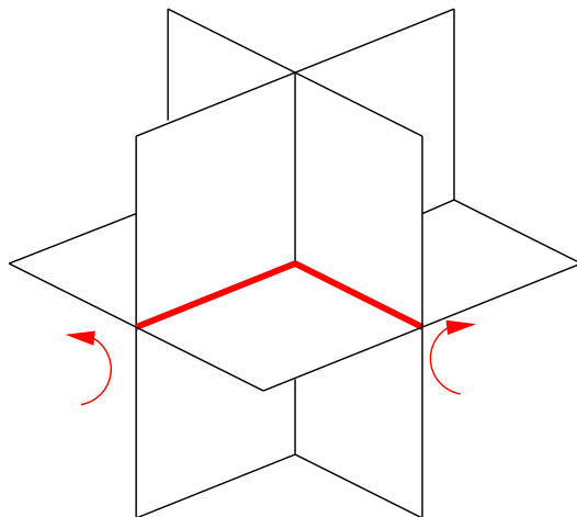
D_{2h}
