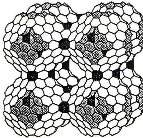
(0, 2)
